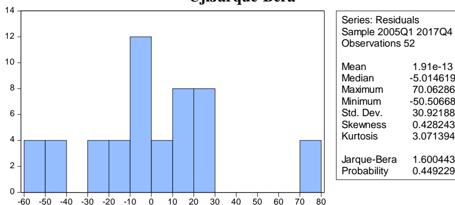
Grafik 4.5 Uji Jarque-Bera
